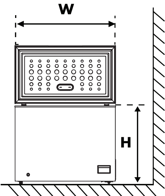
Abbildung 1. Vorderansicht
