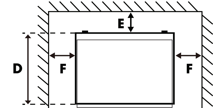
Abbildung 2. Draufsicht
