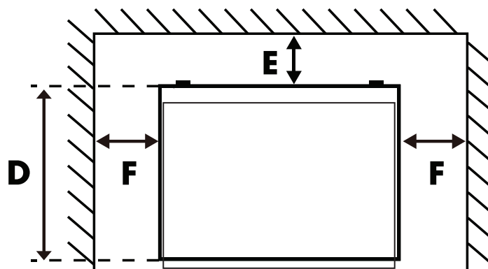
• Figuur 2. Bovenaanzicht
