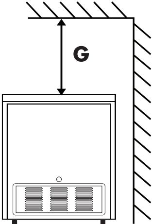
Abbildung 3. Seitenansicht
